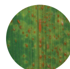
Rouille naine
