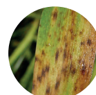
Ramulariose
