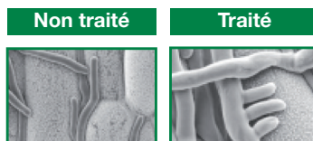
Croissance mycélienne
